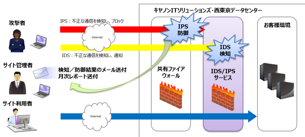
<IDS/IPS サービスのシステム概要図>
