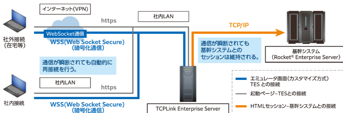
「TCPLink」概要図
